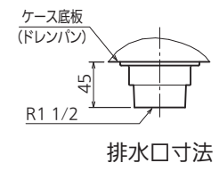
正面図
