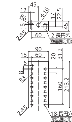
上部振れ止め金具 (同梱部品)
