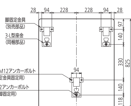
アンカーボルト位置上面透視図 (標準施工2)
