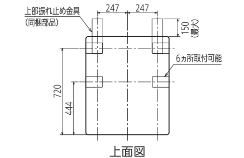
上面図
