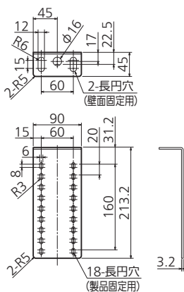
上部振れ止め金具 (別売部品)
