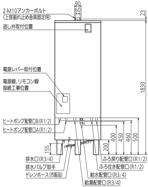
正面図
