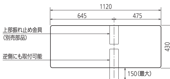
上面図
