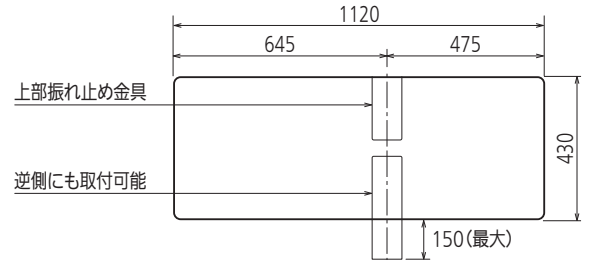
上面図
