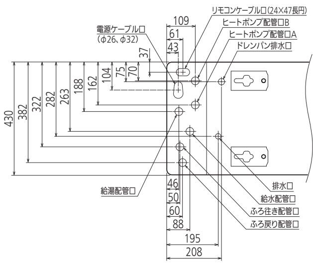
配管位置上面透視図
