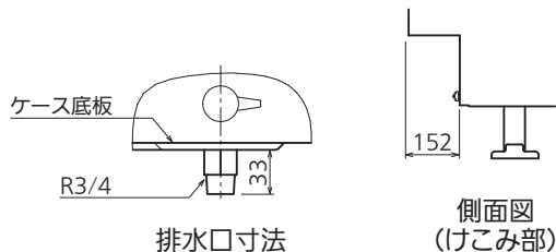
排水口寸法
