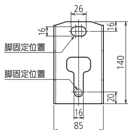
側面図 (けこみ部)
