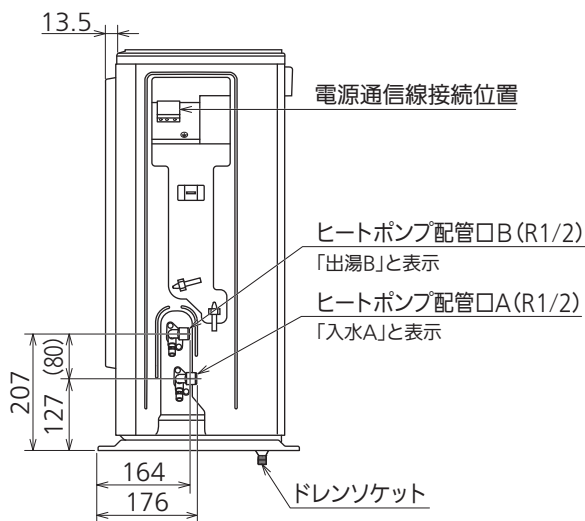
右側面図
