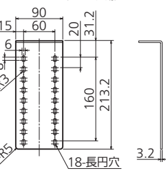
上部振れ止め金具 (同梱部品)
