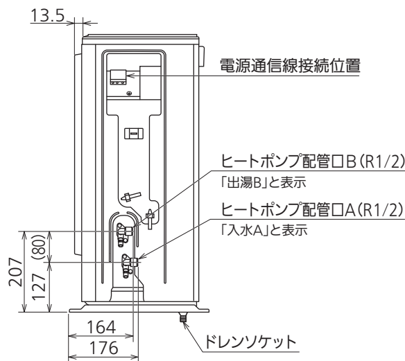
側面図
