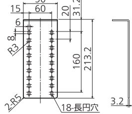
上部振れ止め金具 (同梱部品)
