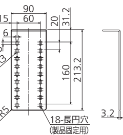
上部振れ止め金具 (同梱部品)
