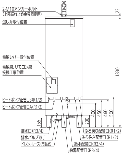
正面図
