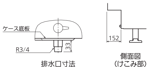
正面図
