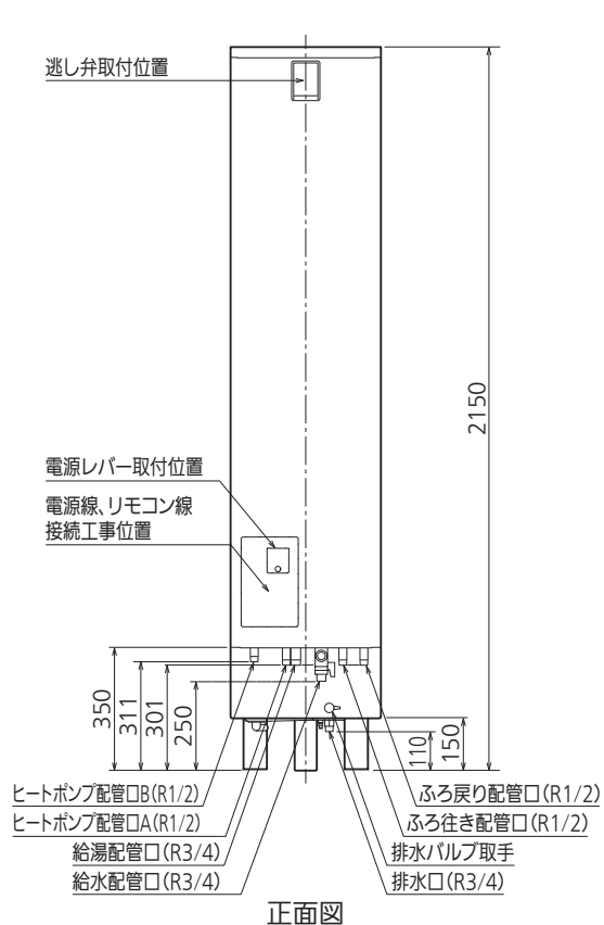
正面図
