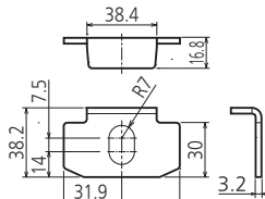
L型座金 (同梱部品)
