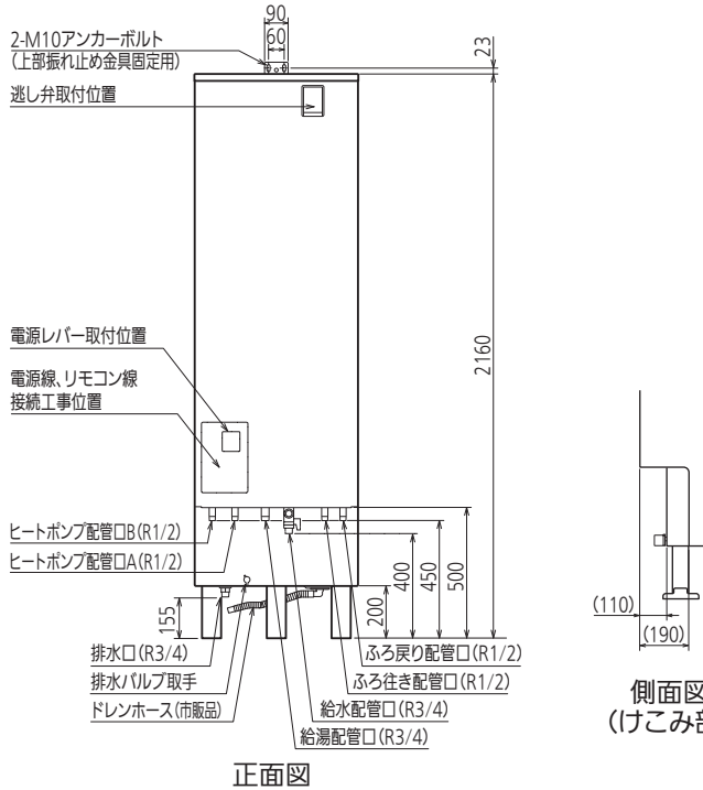
正面図
