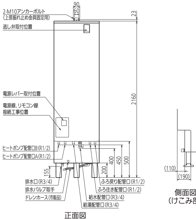
正面図
