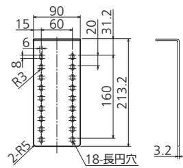
2-長円穴 (壁面固定用)
