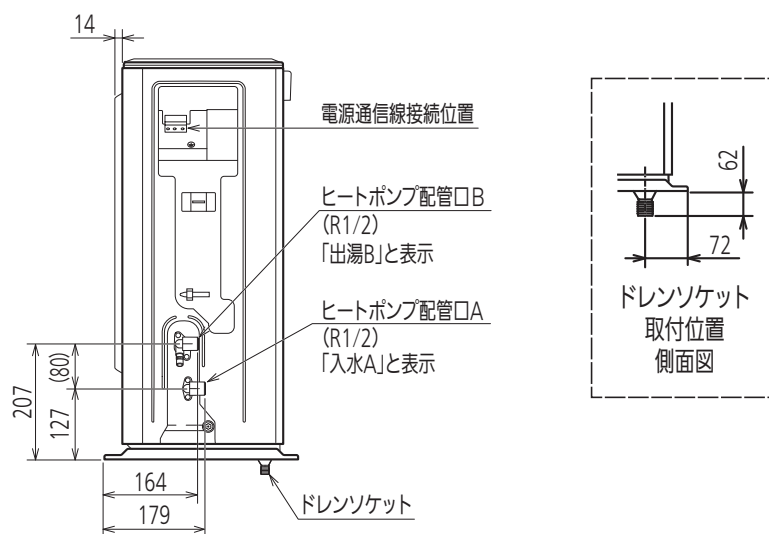
側面図
