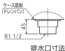
排水口寸法
