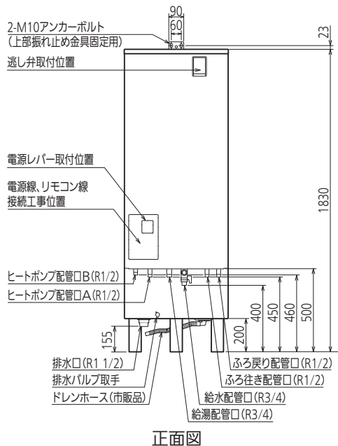
正面図
