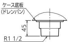
排水口寸法
