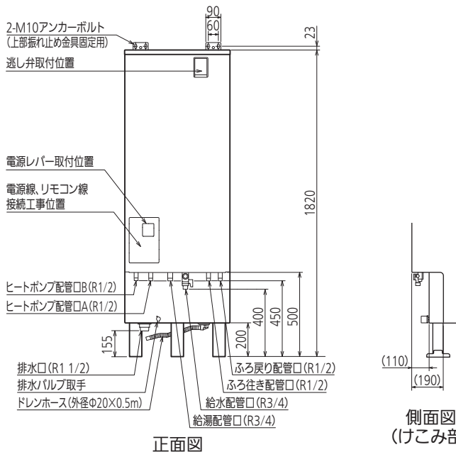
正面図
