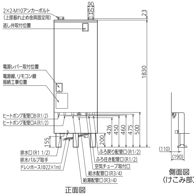
正面図
