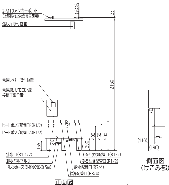
正面図
