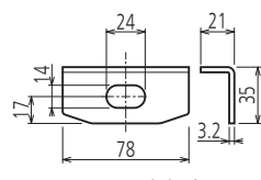
BWL型座金 (同梱部品)
