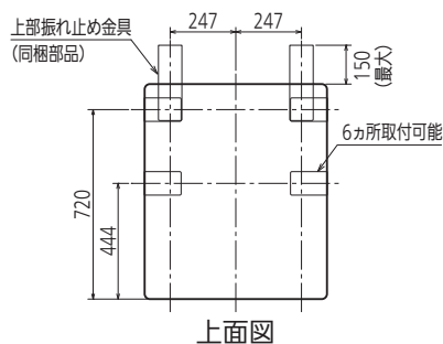
上面図
