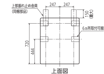
上面図
