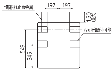
上面図
