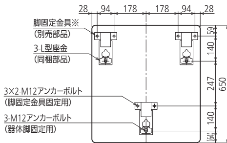
アンカーボルト位置上面透視図 (標準施工2)
