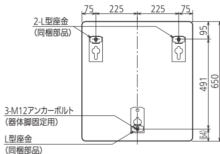
アンカーボルト位置上面透視図 (標準施工1)
