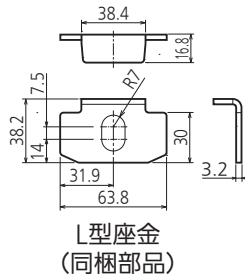
L型座金 (同梱部品)
