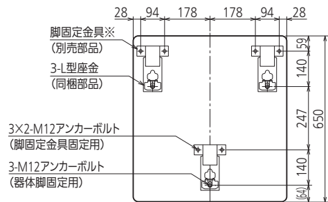
アンカーボルト位置上面透視図 (標準施工2)
