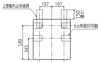
上面図
