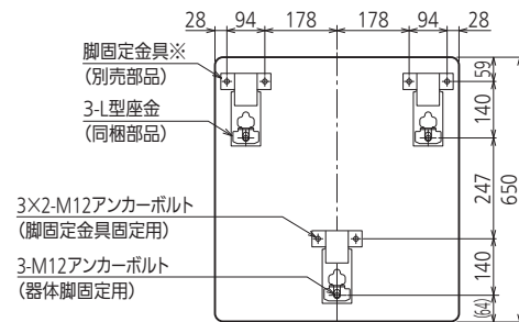
アンカーボルト位置上面透視図 (標準施工ができない場合)
