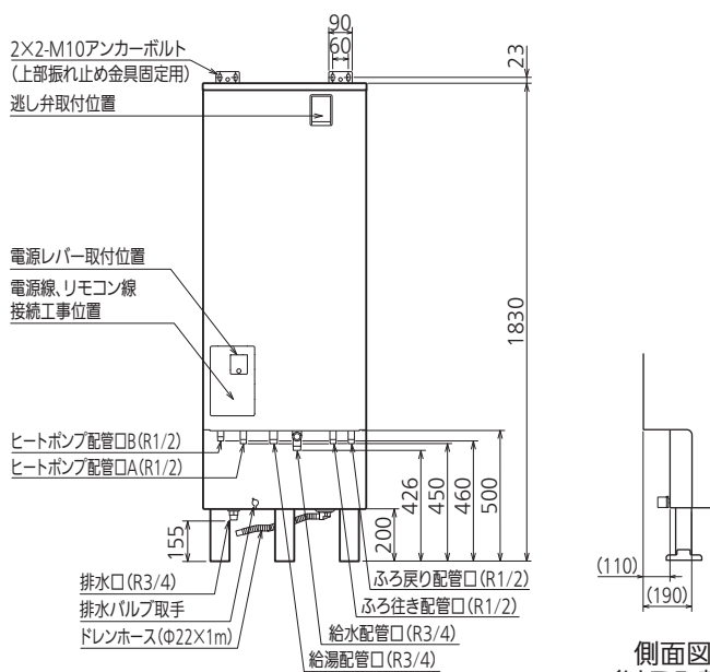
正面図
