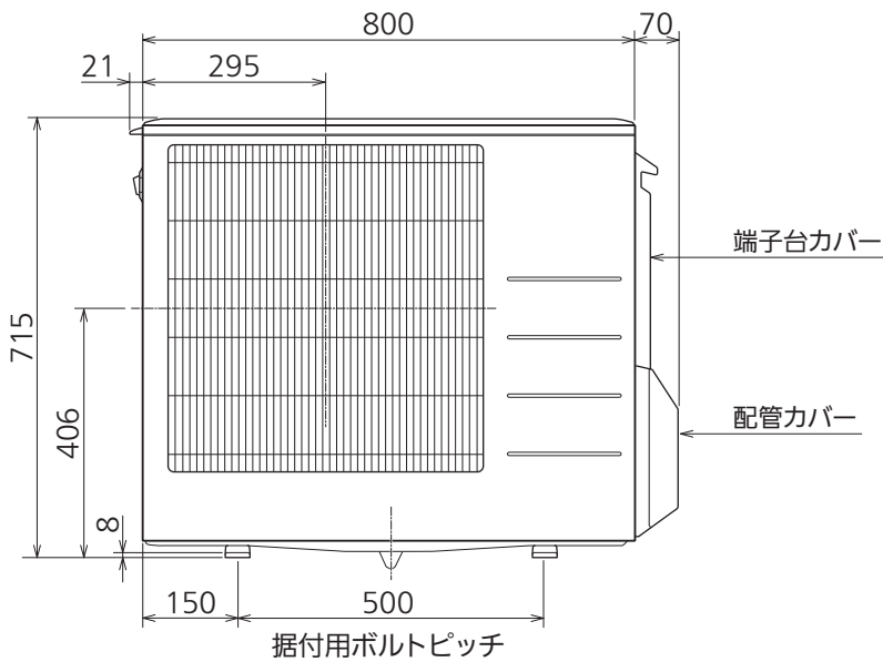
正面図
