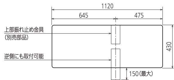
上面図
