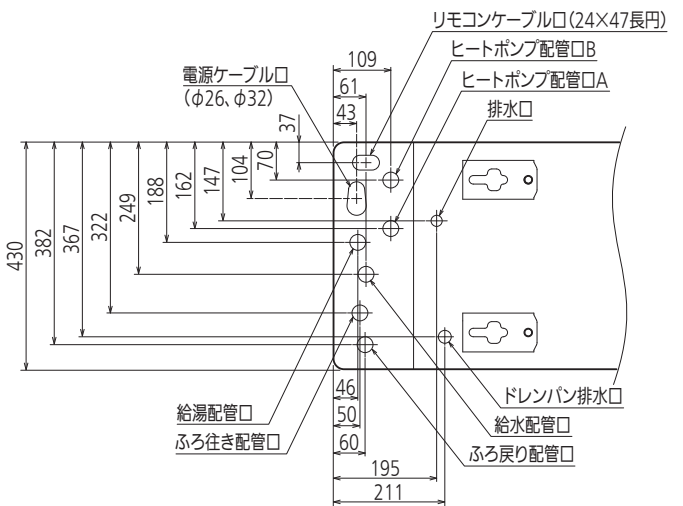
配管位置上面透視図
