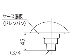
排水口寸法
