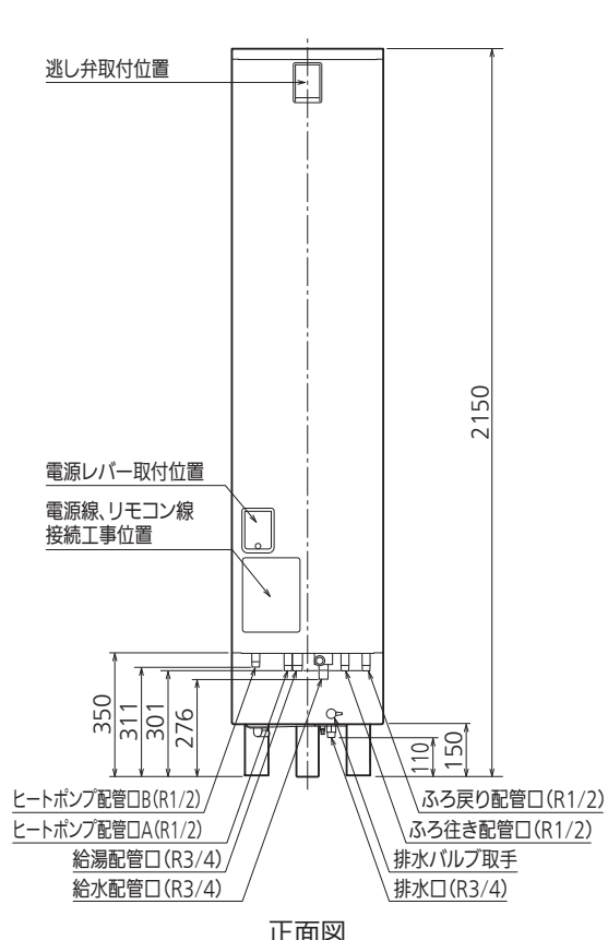
正面図
