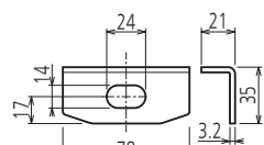
BWL型座金 (同梱部品)
