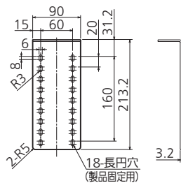
上部振れ止め金具 (同梱部品)
