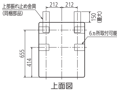
上面図
