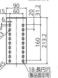
上部振れ止め金具 (同梱部品)
