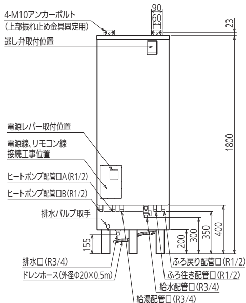
正面図
