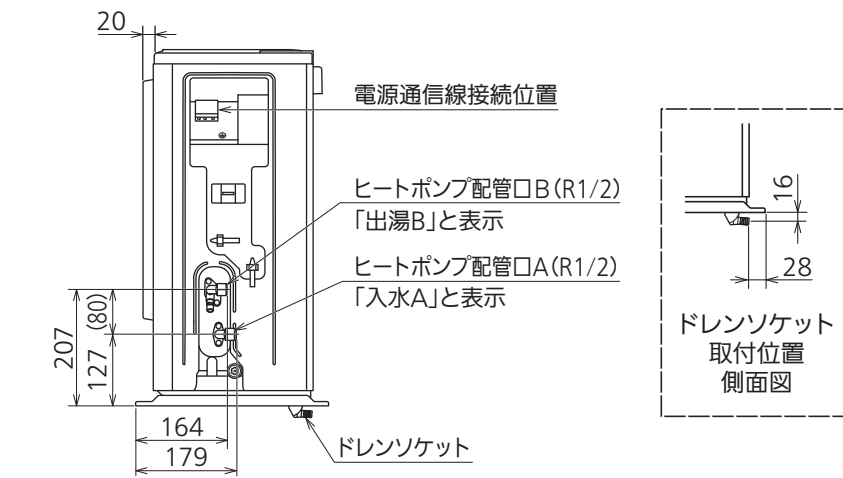
正面図
