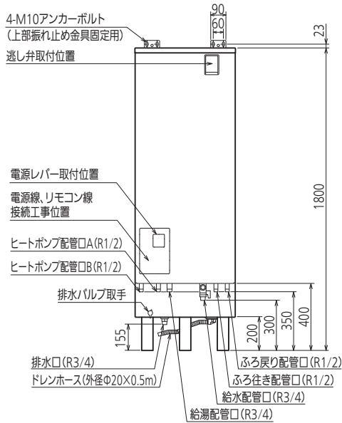
正面図
