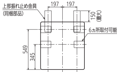
上面図
