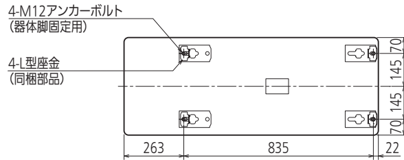
アンカーボルト位置上面透視図 (標準施工時)
