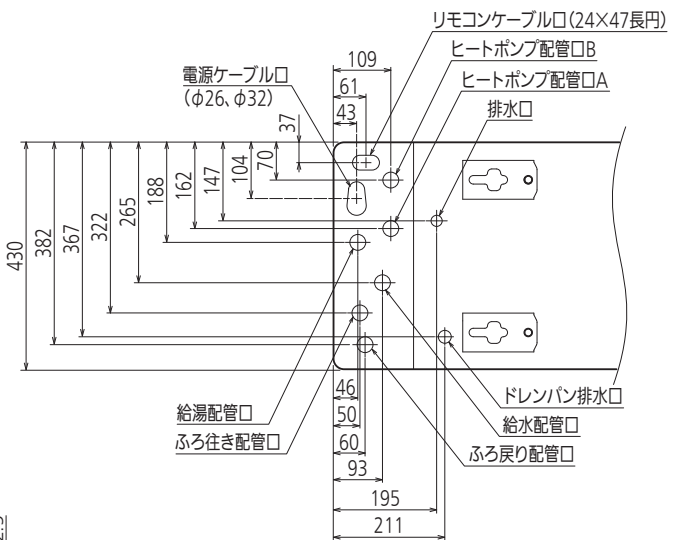
配管位置上面透視図
