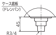
排水口寸法
