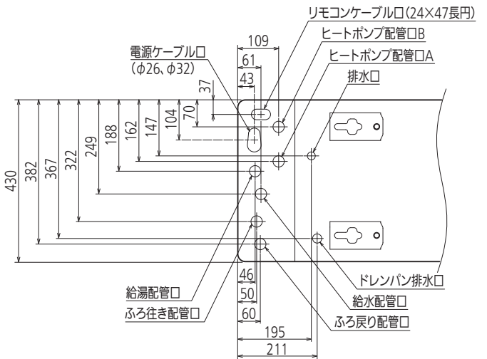
配管位置上面透視図
