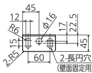
排水口寸法
