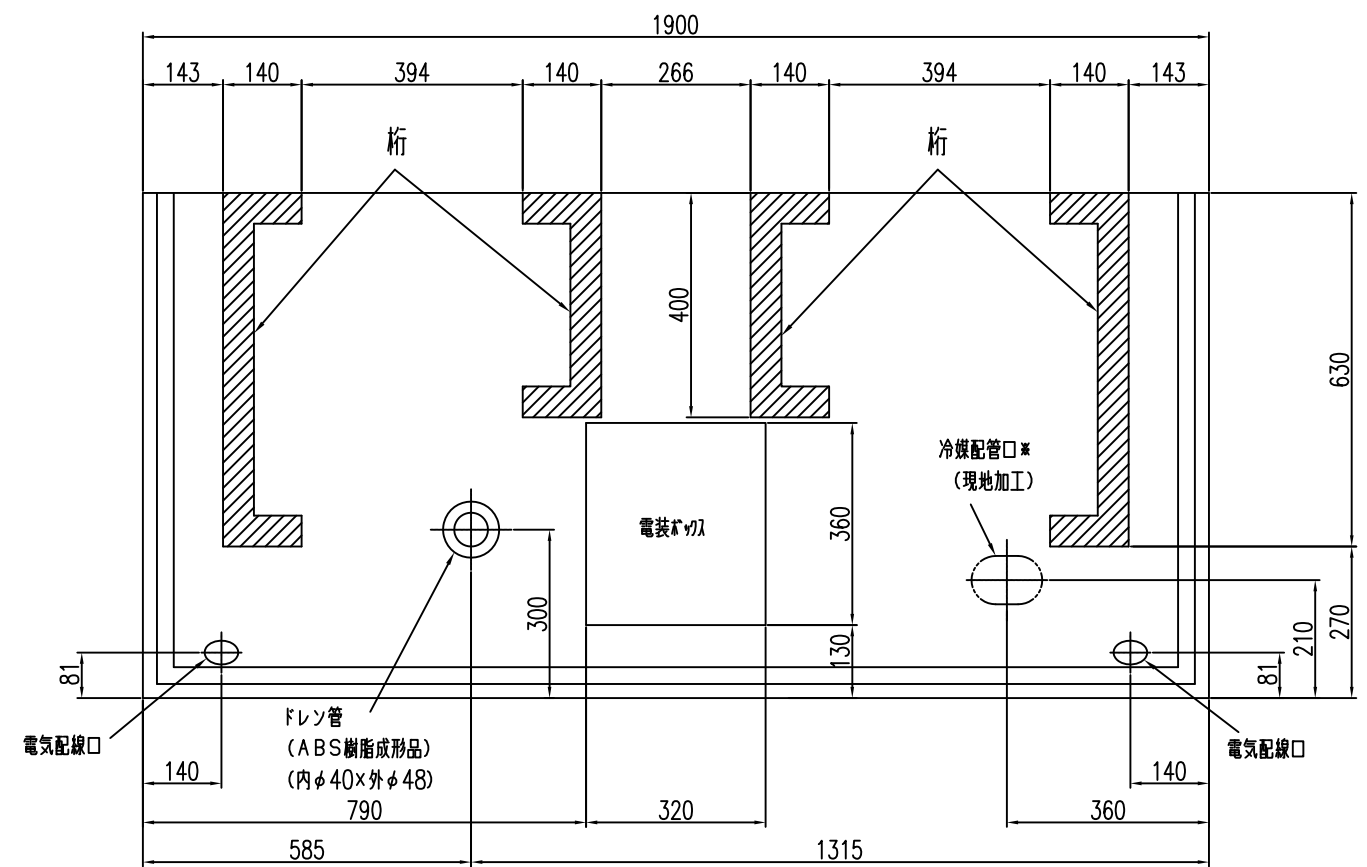
底部平面図
