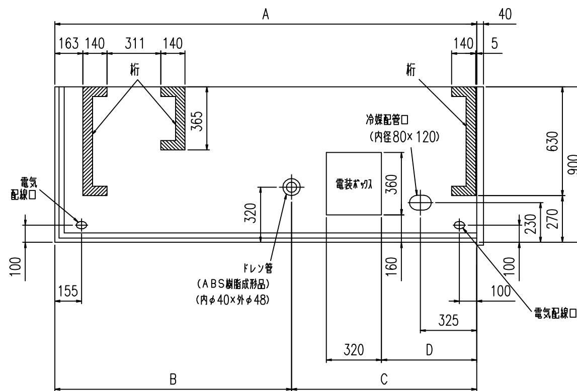
平面図
